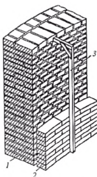
1 – стена ствола трубы; 2 – футеровка; 3 – шаблон для проверки правильности футеровки
