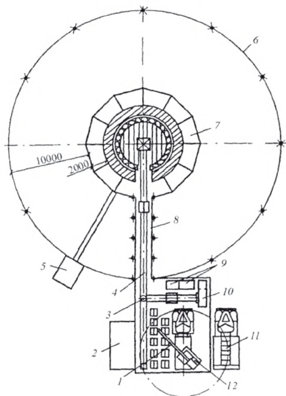
Рисунок Б.19 – Стойгенплан строительства трубы при помощи одношахтного подъемника
