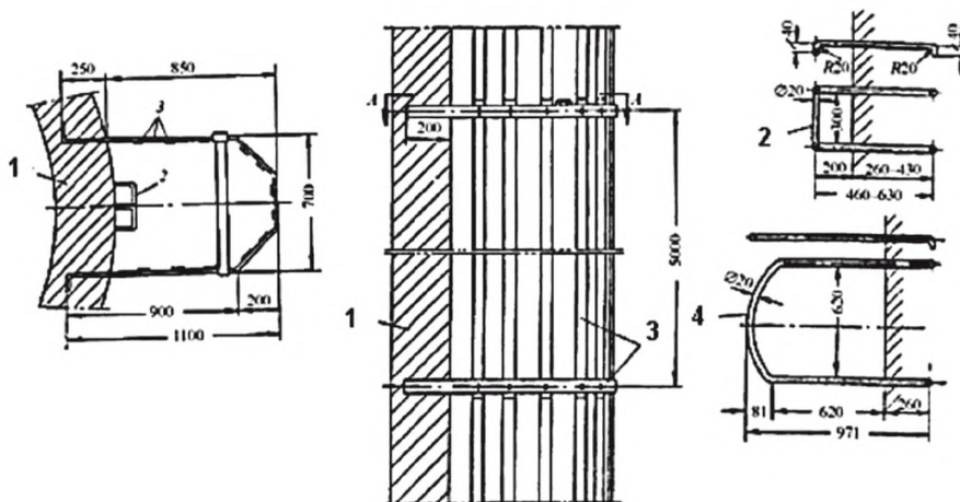
Рисунок 1 – Оголовки труб и защитный колпак
