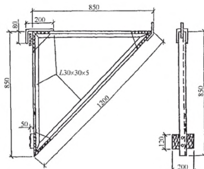
Рисунок 14 – Металлический кронштейн
