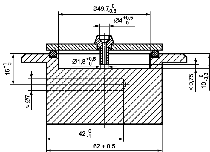
Рисунок А.5 — Поперечное сечение блока через отверстие для ввода пробы
