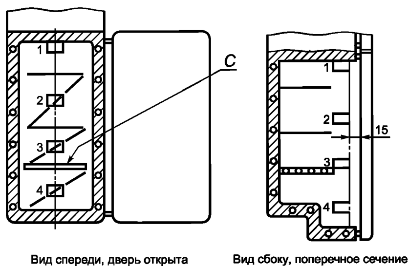
b — Морозильник пищевых продуктов или камера хранения замороженных пищевых продуктов, с неветилируемыми, охлаждающимися стенками или дном, без дверного хранения, с n полками, с естественным ограничением загрузки
