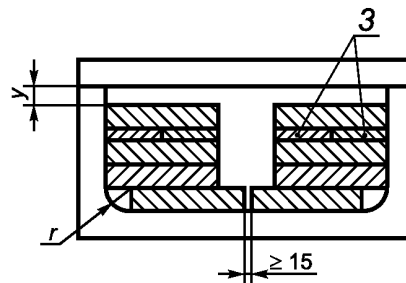
f – Вид спереди с закругленными углами
