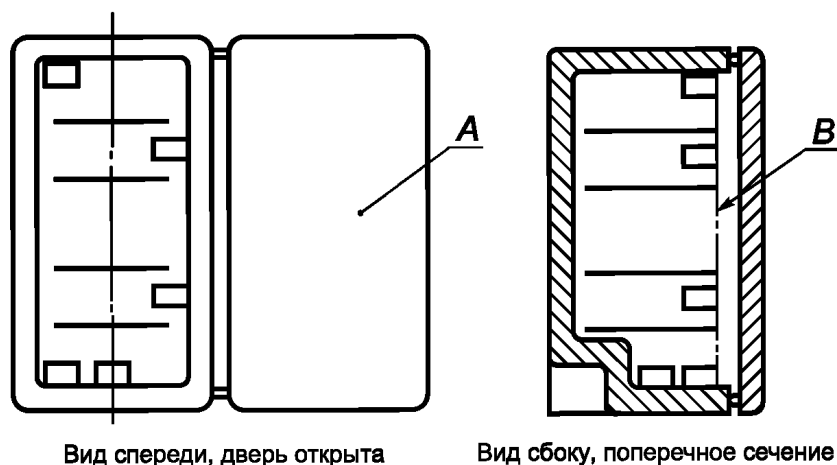
a — Морозильник или шкаф три звезды, без дверного хранения, с n полками, с обозначенной линией допустимой загрузки
