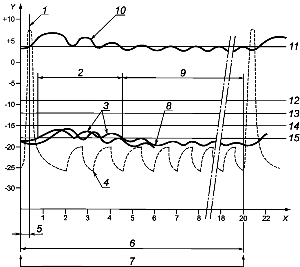
X — время, ч; Y — температура, °C; 1 — начало процесса охлаждения; 2 — период 20 % рабочего цикла максимальной продолжительностью 4 ч, когда допускается повышение температур в М-пакетах в холодильной камере; 3 — моментальные температуры в различных М-пакетах; 4 — температура испарителя; 5 — цикл автоматического оттаивания; 6 — рабочий цикл; 7 — моменты, когда включаются средства оттаивания; 8 — моментальная температура в самом теплом М-пакете; 9 — период, в ходе которого должны выполняться условия таблицы 2, за исключением сноски a) ; 10 — t a ; 11 — t ma ; 12 — t** + 3 К; 13 — t**, 14 — t*** + 3 К; 15 — t***
