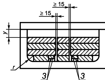
e – Вид спереди с закругленными углами
