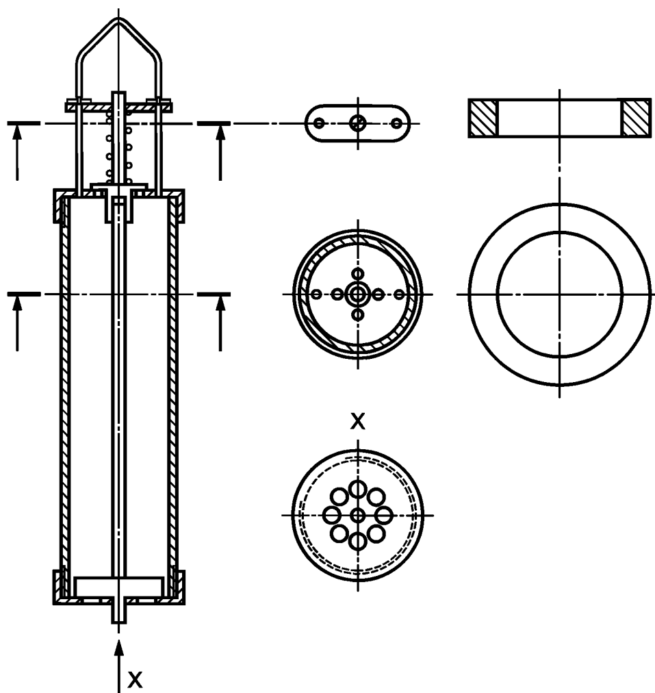
Рисунок В.4 — Донный пробоотборник
