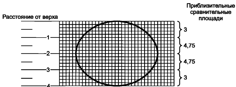
а – Поперечное сечение горизонтального резервуара эллиптической формы
