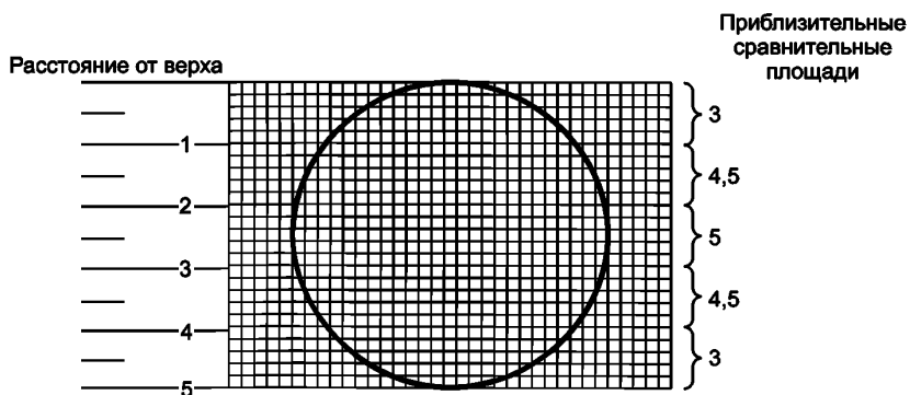
б – Поперечное сечение горизонтального резервуара цилиндрической формы
