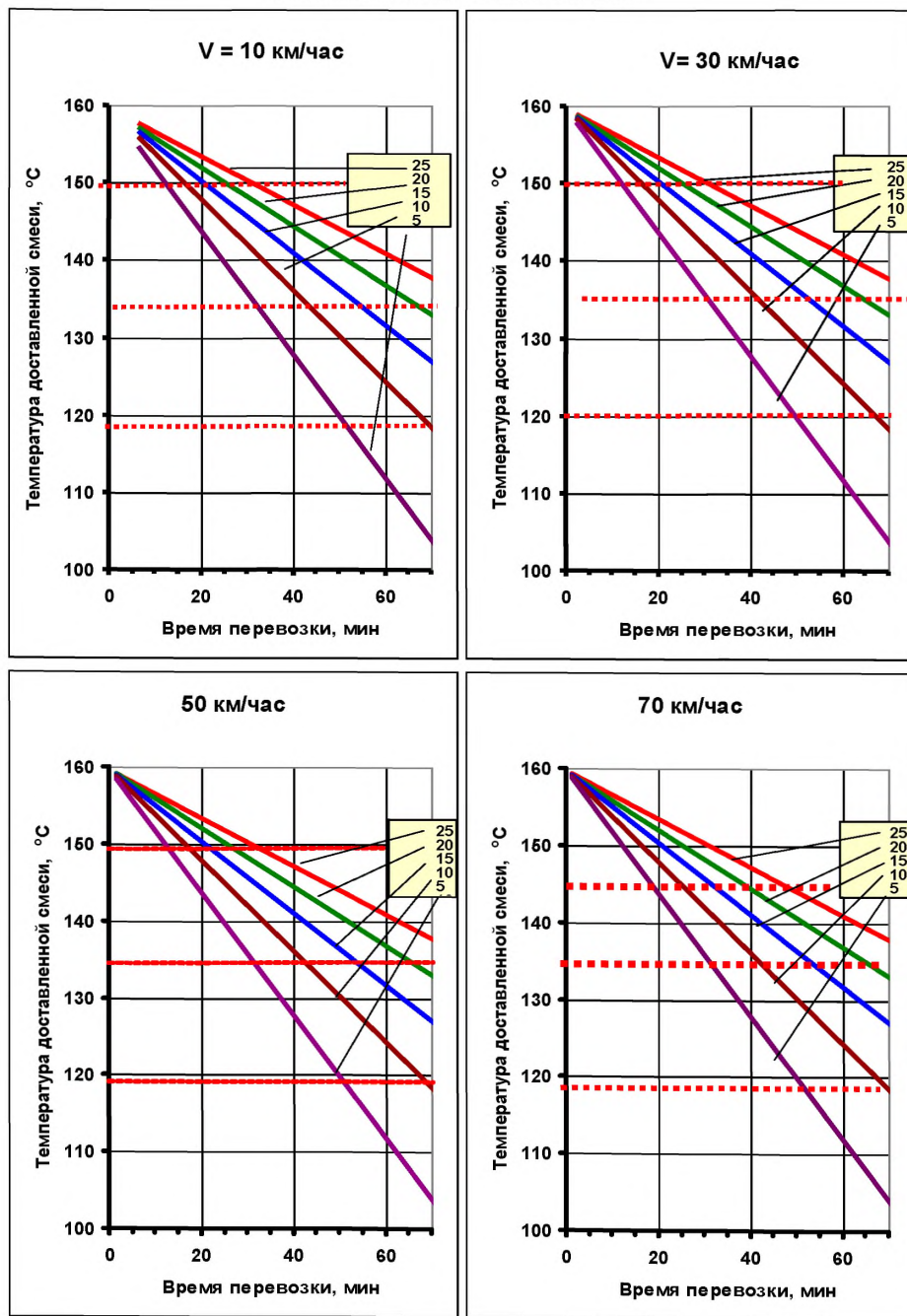
Рисунок В.1 Время перевозки горячей асфальтобетонной смеси в автомобилях самосвалах (при температуре отгрузки t_{\text{нач}} = 160 °C)
