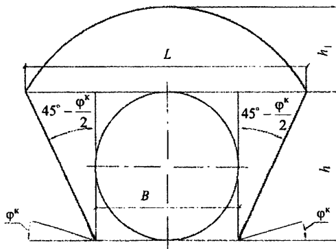
Рисунок 1 – Схема для расчета высоты свода обрушения
