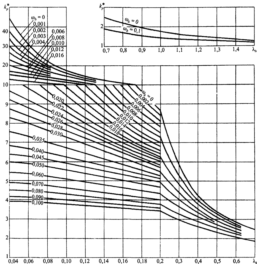
Рисунок 1 – График для определения значений коэффициента k_p^*
