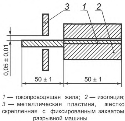
Рисунок 18 — Схема устройства для испытания на адгезию
