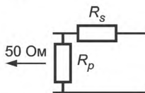
Рисунок 4 — Цепь согласования при Z_k более 50 Ом
