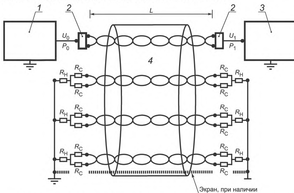
1 — анализатор цепей или генератор сигналов (ГС); 2 — симметрирующий трансформатор; 3 — анализатор цепей или измерительный приемник (ИП); 4 — измеряемый кабель; R_H — резистор несимметричной цепи; R_C — резистор симметричной цепи; L — длина измеряемого кабеля; P_0(U_0) — мощность (напряжение) сигнала на выходе ГС; P_1(U_1) — мощность (напряжение) сигнала на входе ИП
