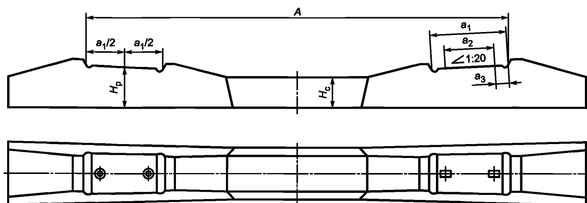
Рисунок 2 — Схема шпал типа III
