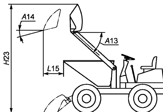
Рисунок 31 — Размеры самозагружающегося мини-землевоза
