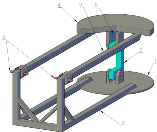
Рис. 10.1. Конструкция стенда, предназначенного для определения параметров воздействия установок динамического нагружения.
