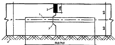
1 – штыревое соединение; 2 – герметизирующий материал; 3 – шпунт; 4 – слой основания
