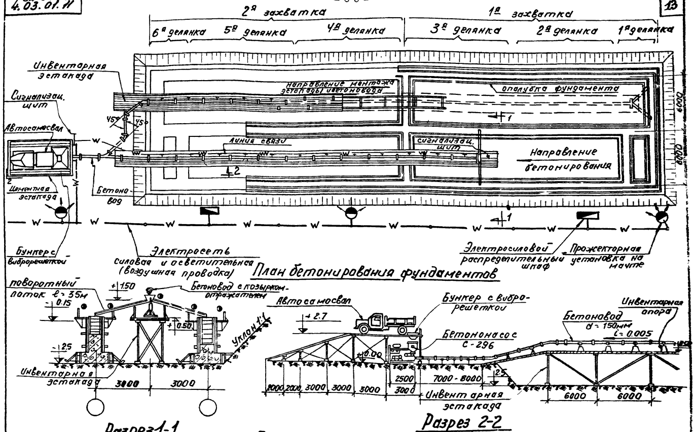
Разрез 1-1
