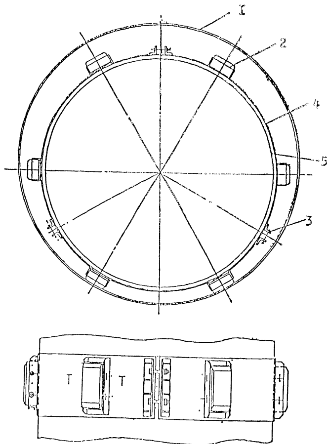
Рис.1. Опорно-направляющее кольцо:
