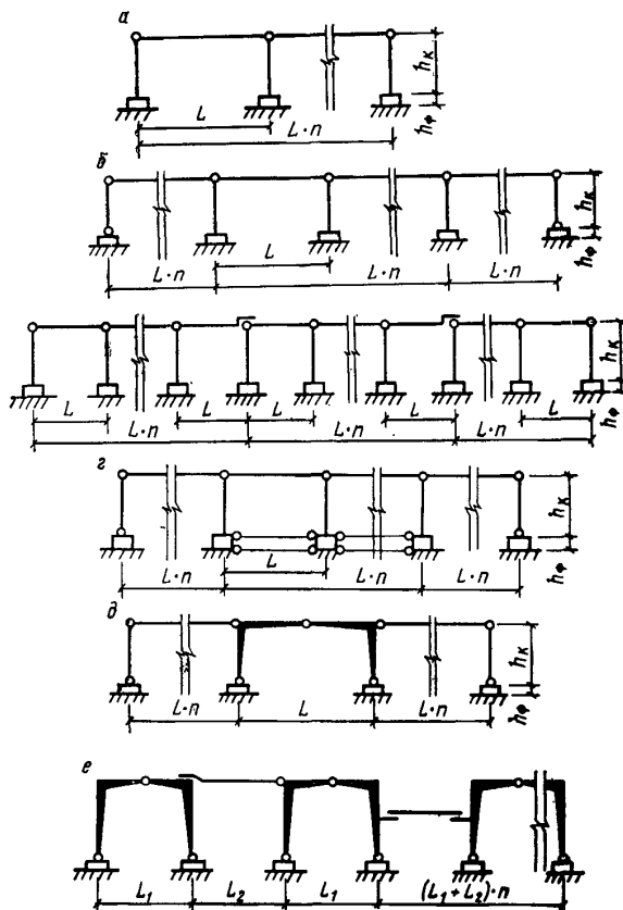
Рис. 5. Схемы поперечных рам одноэтажных каркасных зданий
