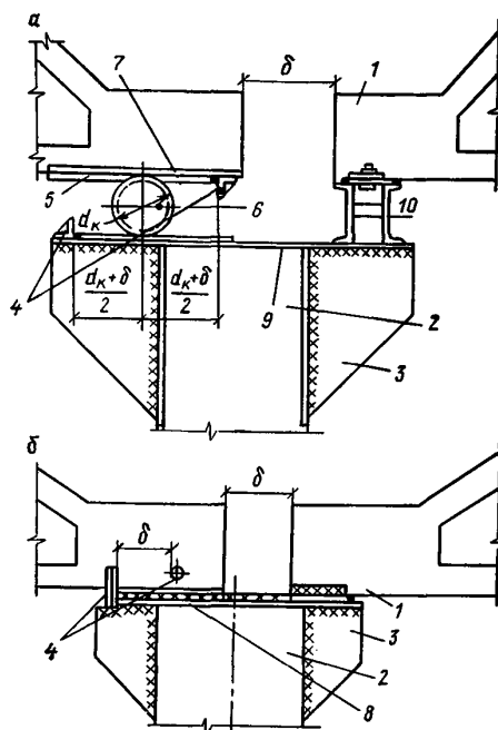
Рис. 7. Шарнирно-подвижные соединения
