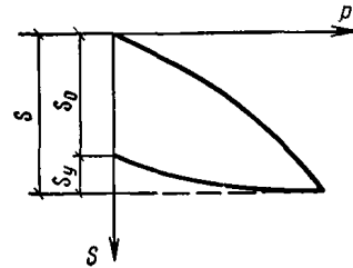
Рис. 2. Зависимость осадки от давления при штамповых испытаниях
