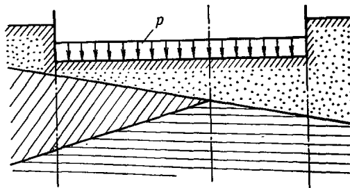
Рис. 1. Геологический разрез неоднородного основания
