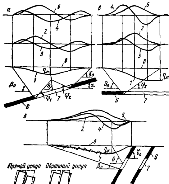
Рис. 1. Механизм движения и эпюры деформаций земной поверхности
