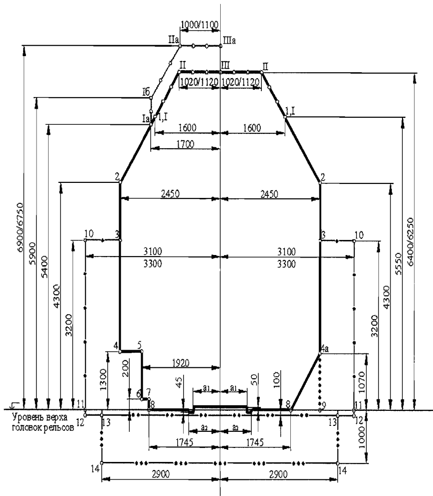
Рисунок 1 - Габарит С 250
