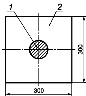
1 — цилиндрический индентор; 2 — образец для испытания
