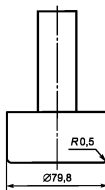
Рисунок 3 — Цилиндрический индентор
