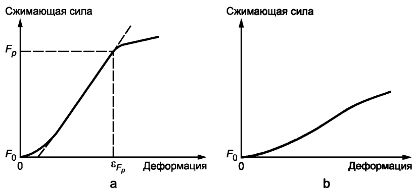
Рисунок 4 — Примеры кривых зависимости деформации от силы
