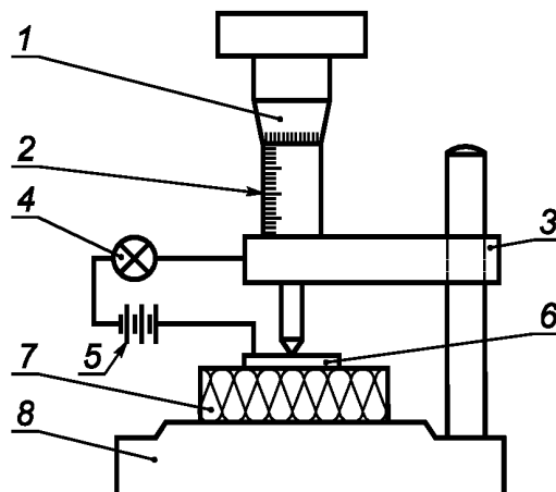
1 — винтовой микрометр; 2 — шкала с делениями в миллиметрах; 3 — регулируемая опора; 4 — лампа; 5 — батарея; 6 — алюминиевая пластина площадью 10 \text{ см}^2 ; 7 — образец для измерения; 8 — основание
