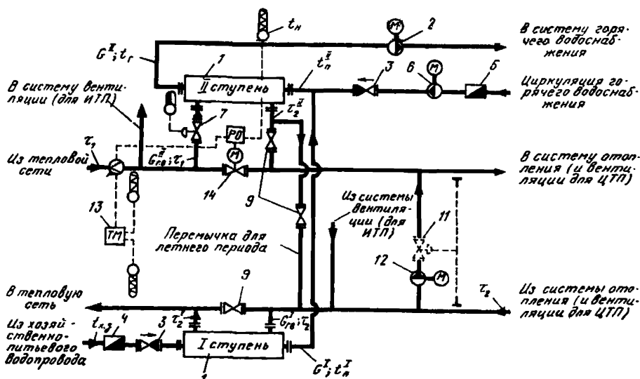
Рис. 6. Двухступенчатая последовательная схема присоединения водонагревателей горячего водоснабжения при применении регулятора изменения расхода воды на вводе по температуре наружного воздуха с зависимым присоединением системы отопления
