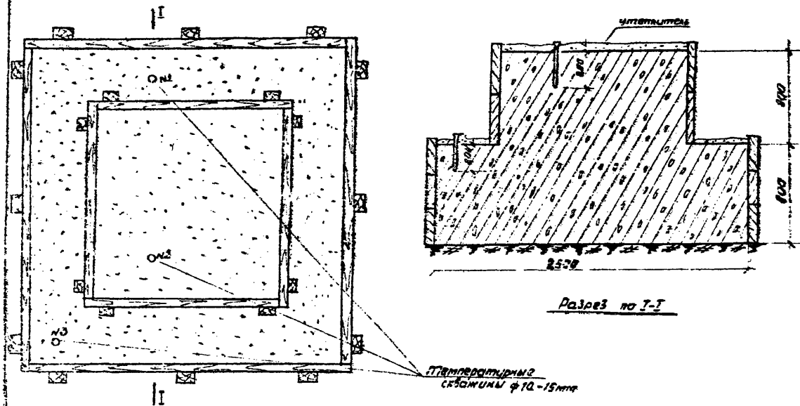
Рис. 2 Расположение и нумерация температурных скважин при электропрогреве танталитовых фризаментав
