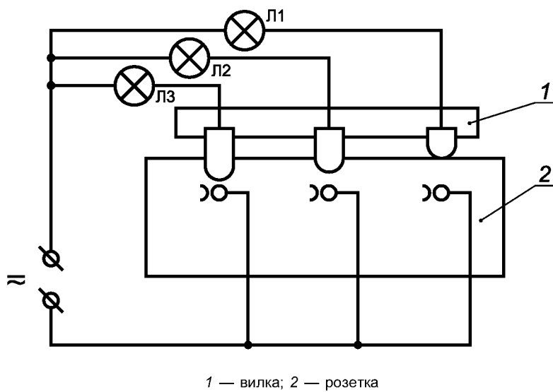
Рисунок ДА.5 — Схема для проверки соединителей с заземляющим контактом на опережающее включение заземляющего контакта
