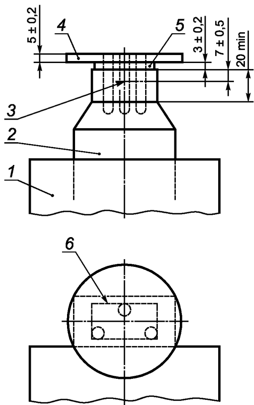
Рисунок 40 — Установка для испытания опрессованных вилок с частично изолированными штырями
