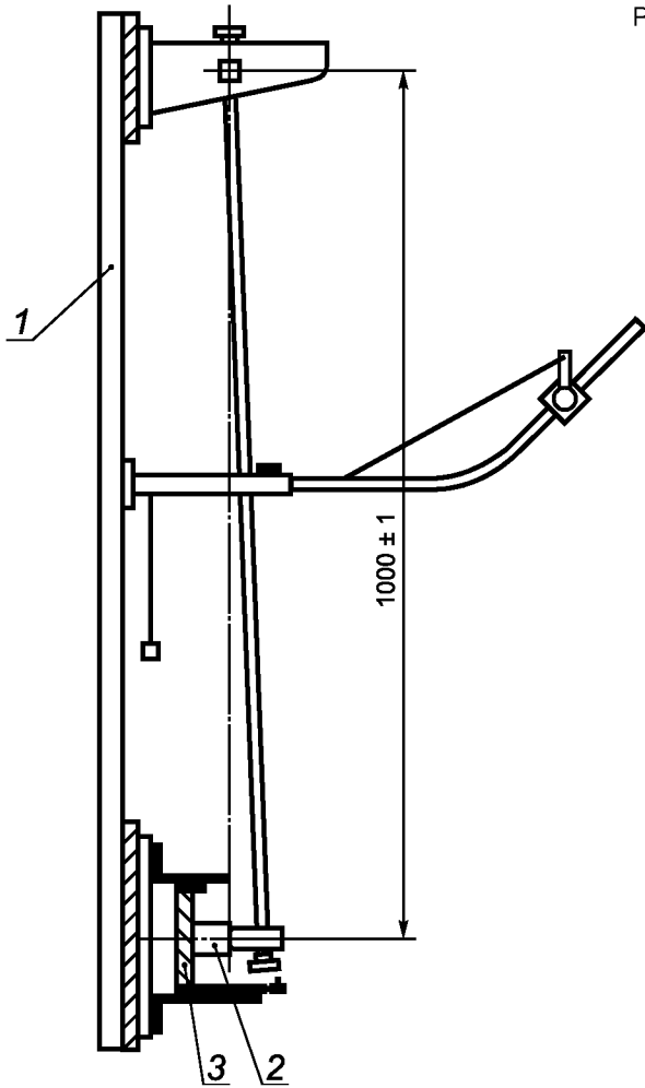
1 — плита; 2 — образец; 3 — монтажная опора
