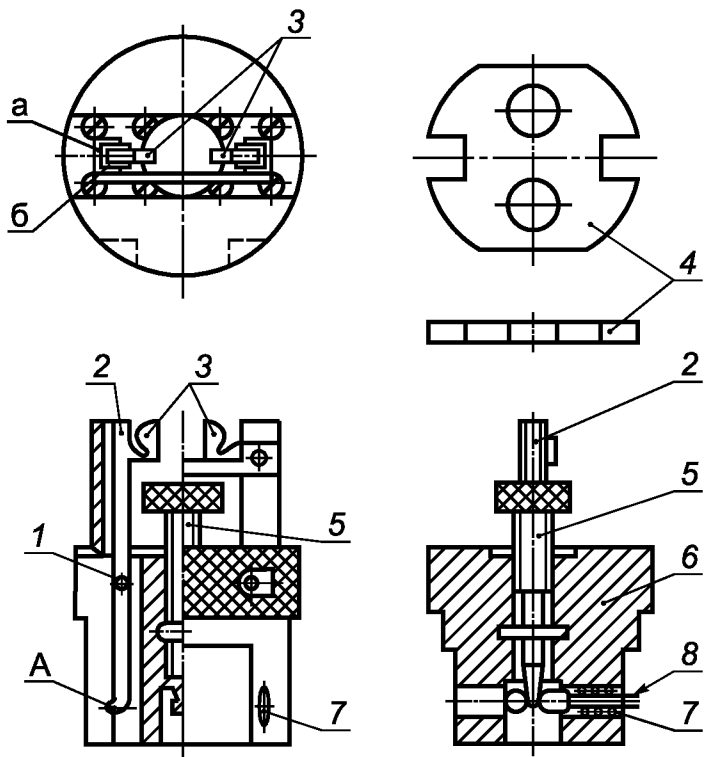
Рисунок ДА.10 — Установка для проверки усилия контактного нажатия боковых заземляющих контактов двухполюсных розеток на 10 и 16 А, 250 В
