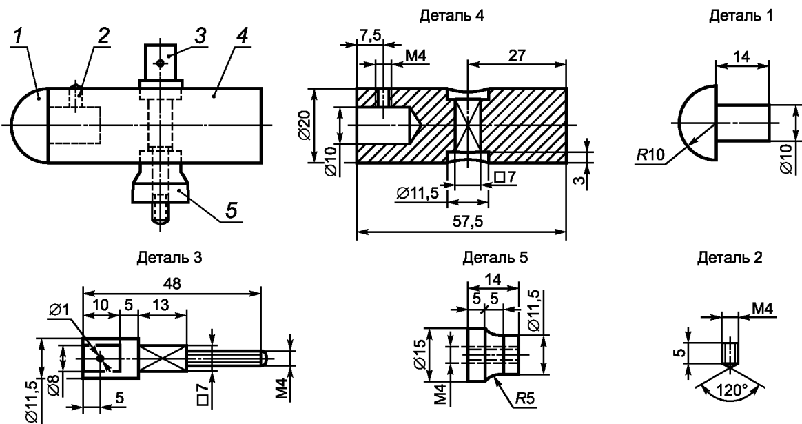
Рисунок 23 — Ударный элемент
