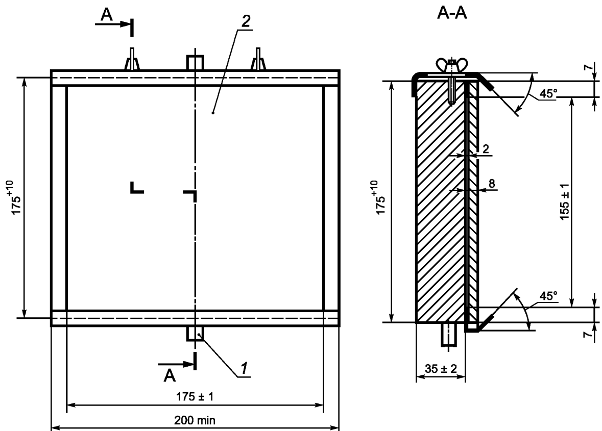
Рисунок 24 — Монтажная опора
