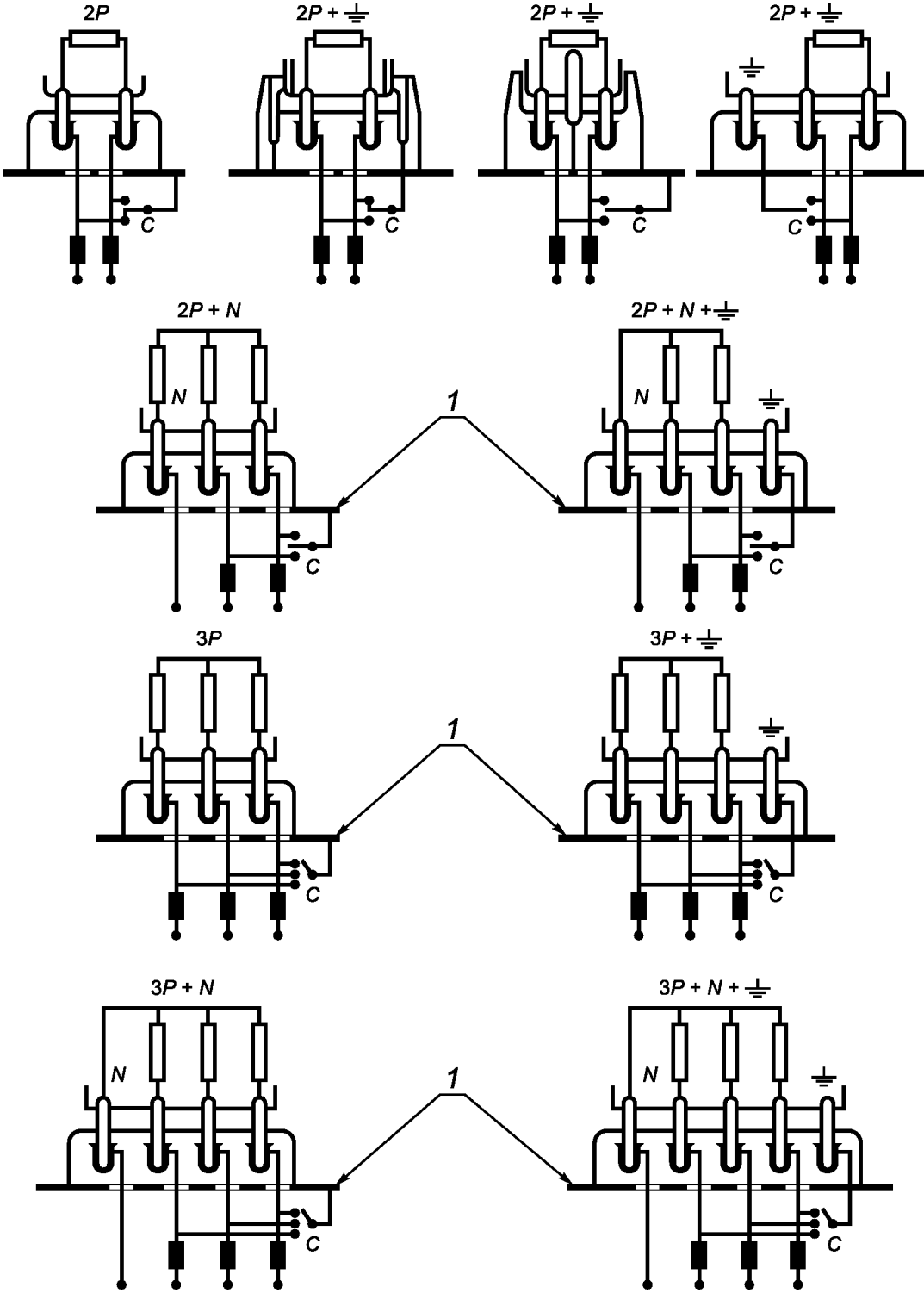
1 — металлическая опора
