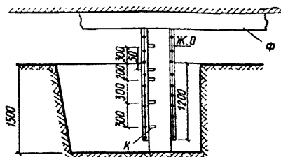
Ф — фундаментные балки; К — место взятия керна; Ж. О — железобетонная обойма усиления фундамента
