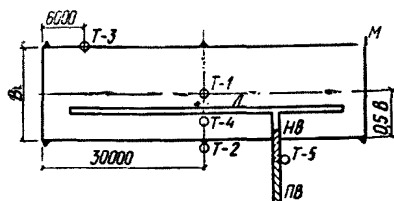
Рис. 1. Расположение температурных скважин и нивелирных марок
