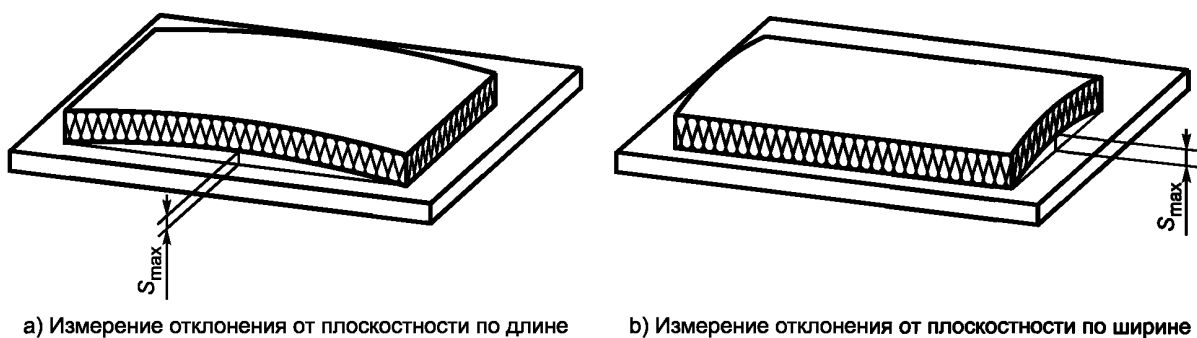
Рисунок 1 — Измерение отклонения от плоскостности
