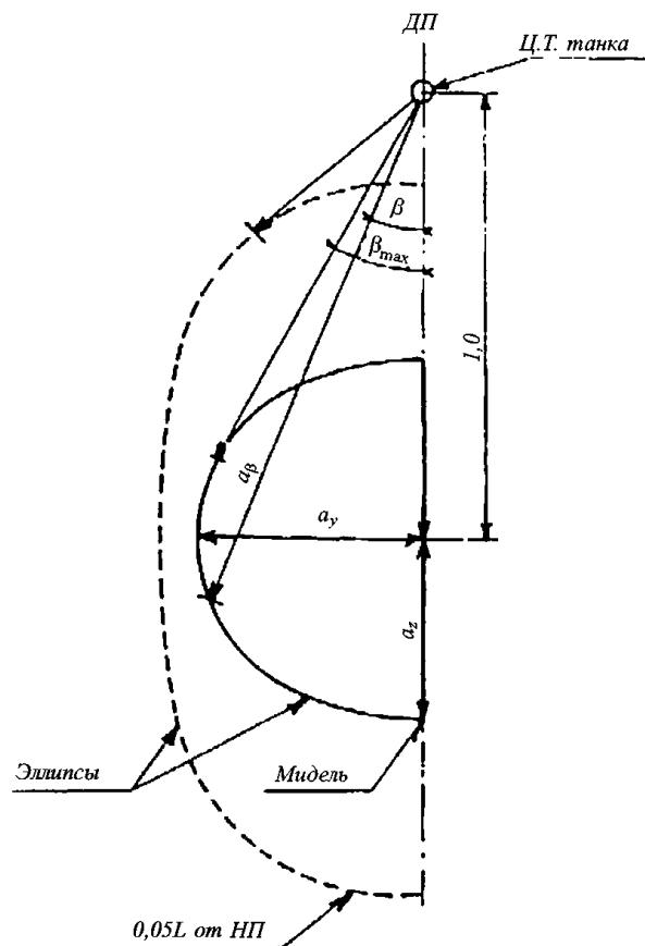
Рис. 3.2-1 Эллипсы ускорения
