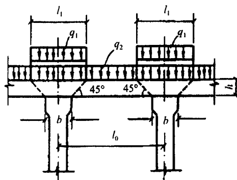
Рисунок 10 – Передача нагрузки от балки на колонну
