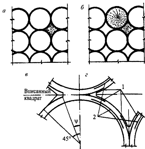
a – загрузка звездочки; б – загрузка звездочки и силоса; в – определение угла \psi ; г – дополнительное армирование стен звездочки; д – опорная арматура; 2 – пролетная арматура
