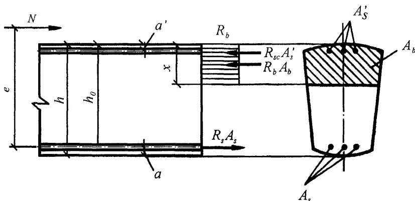
Рисунок 3 – Схема усилий и эпюр напряжений в сечении, нормальном к продольной оси внецентренно сжатого железобетонного элемента, при расчете его по прочности
