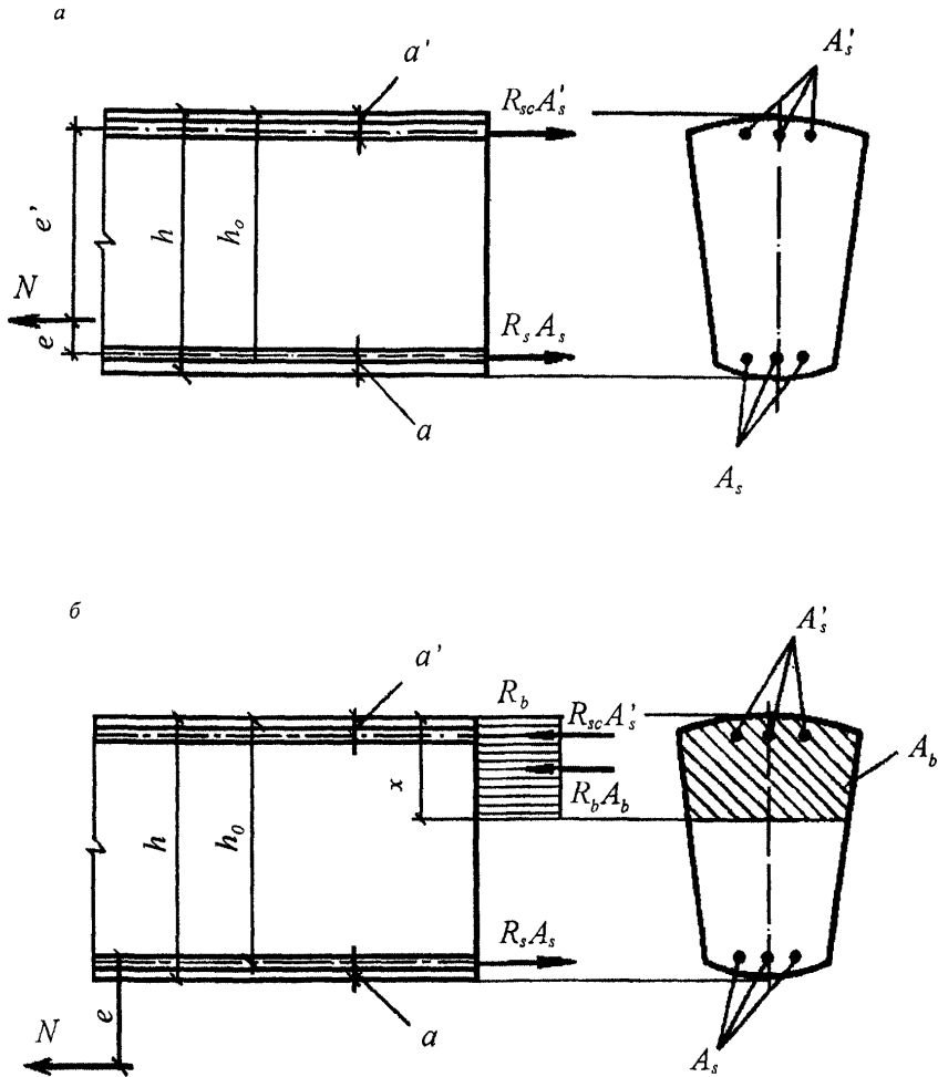
а – продольная сила N приложена между равнодействующими усилий в арматуре A_s и A'_s ; б – продольная сила N приложена за пределами расстояния между равнодействующими усилий в арматуре A'_s и A'_s
