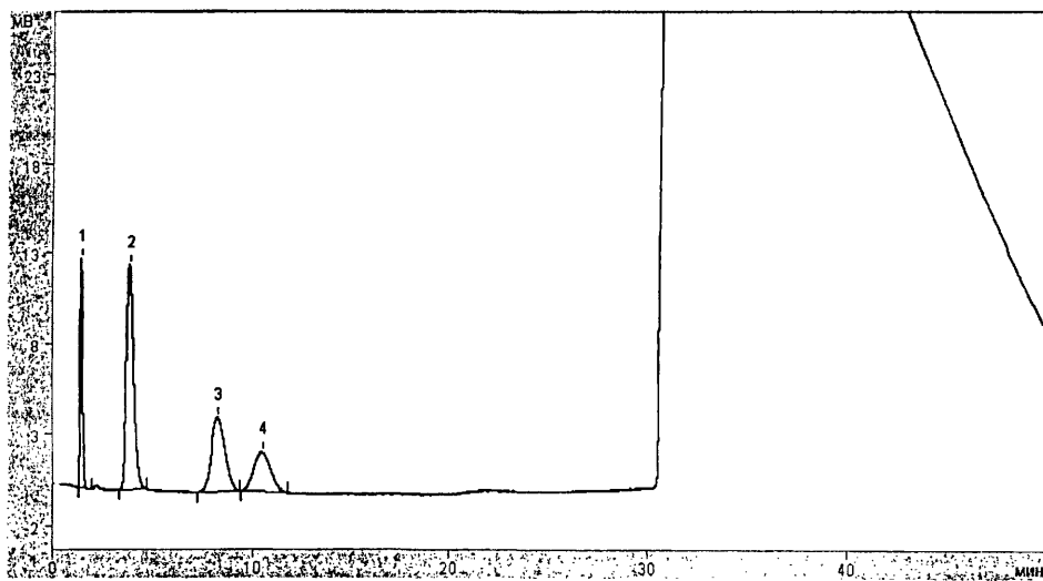
Рис. 2. Хроматограмма градуировочной смеси альдегидов в ДМФА
