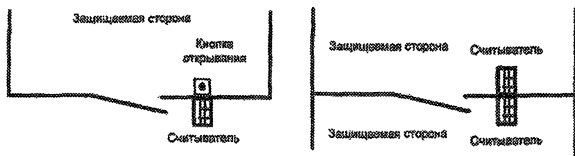
Размещение считывателей на стене
