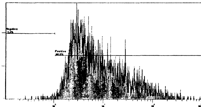
Рис. 7. Пример гистограммы распределения нейтрофилов, стимулированных E. coli (интервал «Positive»), и нестимулированных образцов (интервал «Negative») по интенсивности флуоресценции на канале FL1. Ось ординат — число клеток; ось абсцисс — флуоресценция, отн. ед. Индекс стимуляции рассчитывают как соотношение числа клеток в интервалах «Positive» и «Negative»
