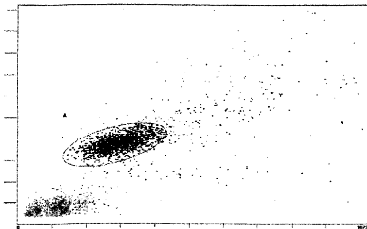
Рис. 8. Пример выделения гейта лимфоцитов (эллипс) на двух каналах светорассеяния: FS Lin и SS Lin. Ось ординат – размер клеток, отн. ед, ось абсцисс – гранулярность, отн.ед.
