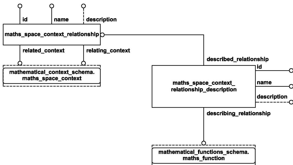
Рисунок D.5 — EXPRESS-G диаграмма схемы mathematical_description_of_distribution_schema (диаграмма 3 из 3)
