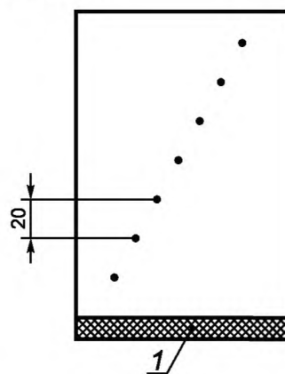
Рисунок С.1 — Нитевидный тест-объект для измерения LSF
