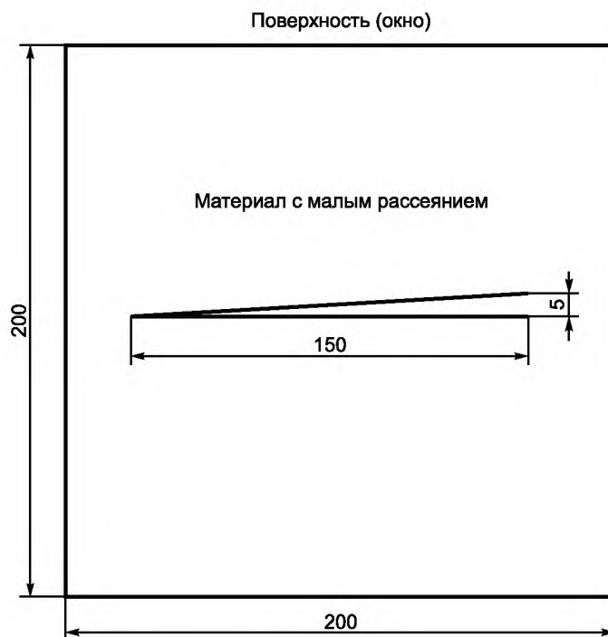
Рисунок С.2 — Тест-объект для оценки осевого разрешения
