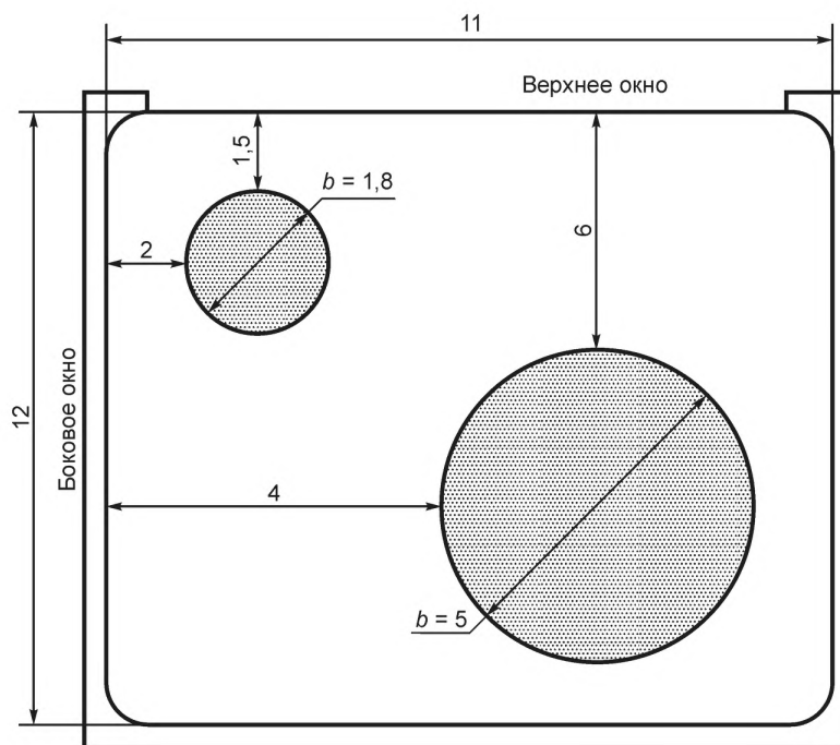
Рисунок В.2 — Композиция изображений двух поперечных сечений мишеней, показанных на рисунке В.1. Вид через боковое окно
