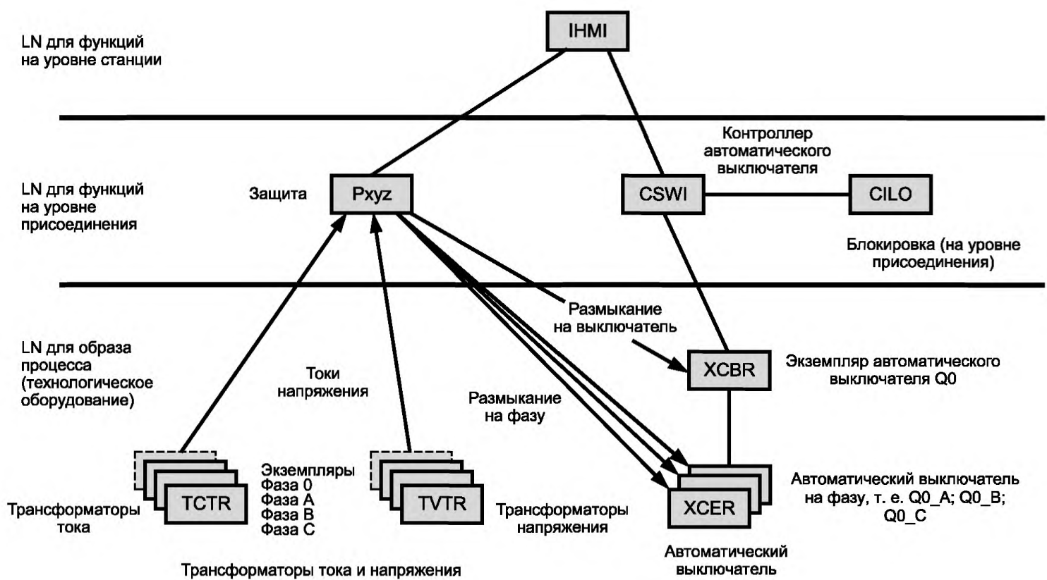
Рисунок 14 — Регулируемый выключатель на фазу (один экземпляр XCER на фазу) и измерительные трансформаторы с аппаратурой измерения на фазу (один экземпляр TCTR или TVTR на фазу)
