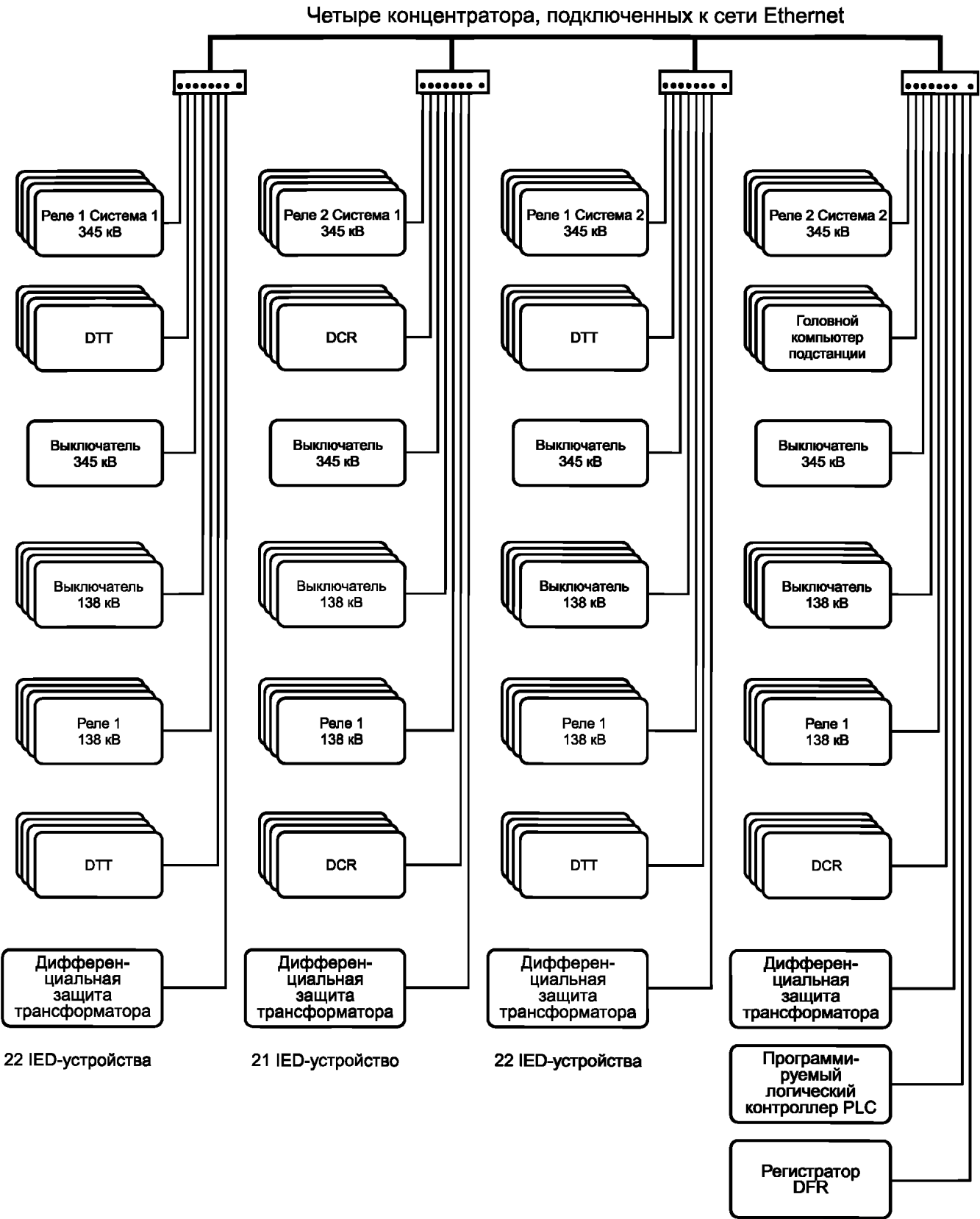
Рисунок I.10 — Конфигурация сети Ethernet с коммутируемым концентратором
