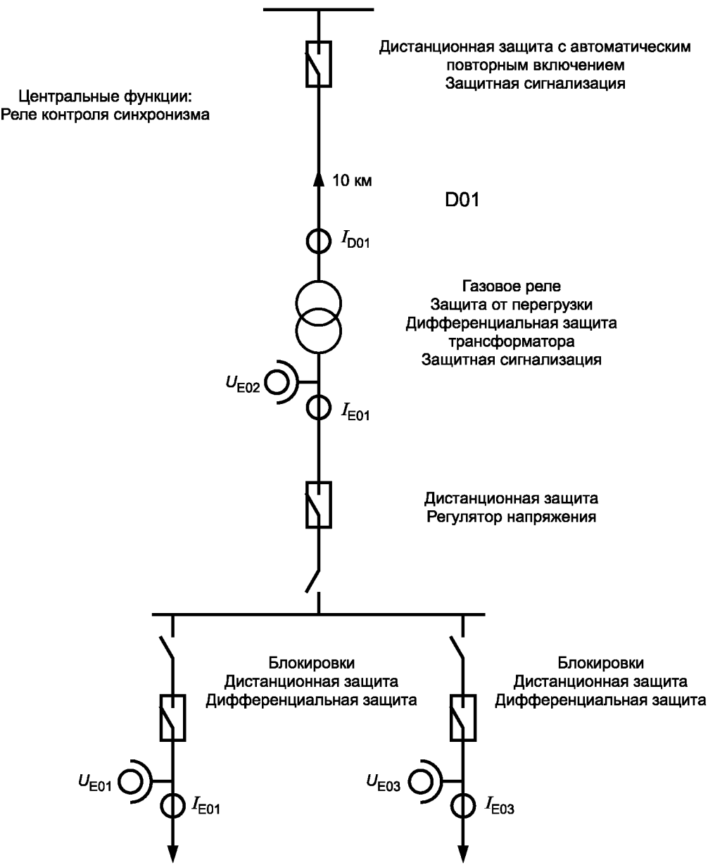
Рисунок I.3 — Подстанция типа Т1-1 с распределением функций
