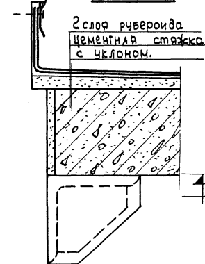
Узел "Е"
