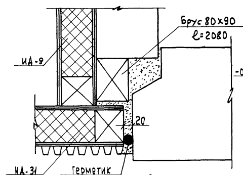
Узел "З"
