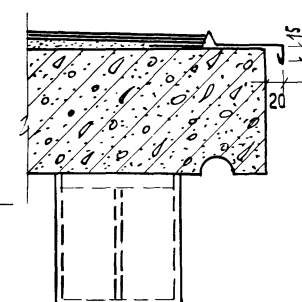
Узел "Ж"
