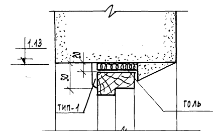
Узел "Г"
