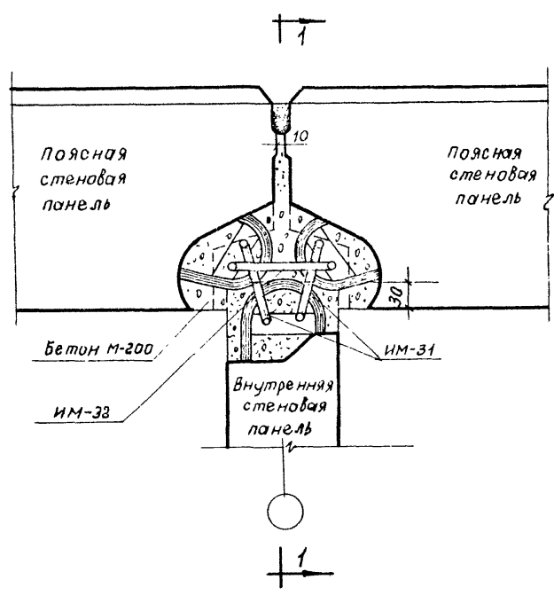
Вертикальный стык
