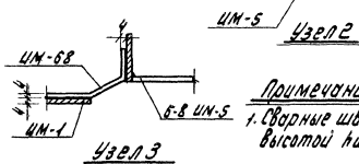
Узел 3
