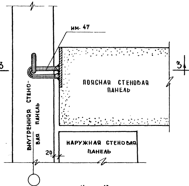
Узел.1
