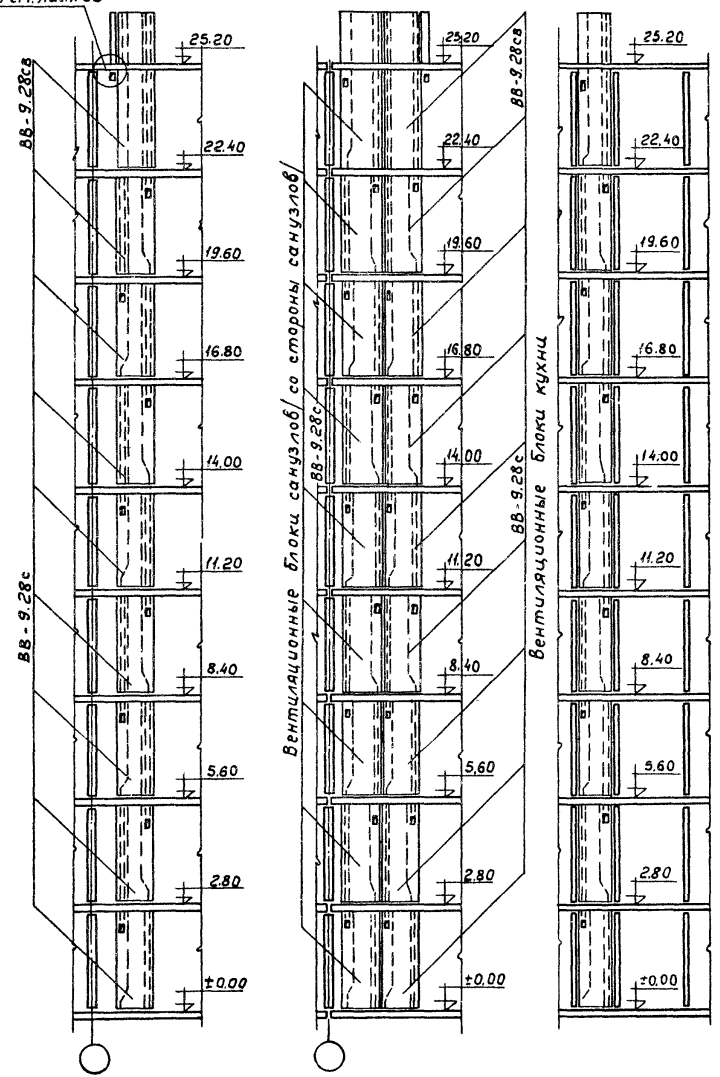
По 1-1 По 2-2 По 3-3 Развертки вентиляционных каналов 5 ти этажных домов
