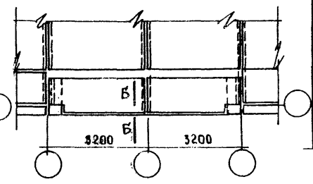
ФРАГМЕНТ МОНТАЖНОГО ПЛАНА И ПЛАНА ПЕРЕКРЫТИЙ (ВАРИАНТ МЕТАЛЛИЧЕСКОГО ОГРАЖДЕНИЯ)
