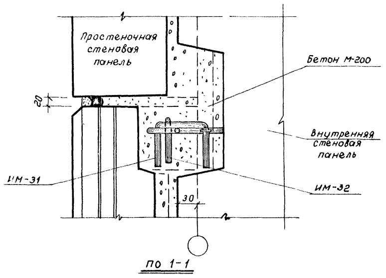
Горизонтальный стык
