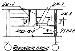
Фрагмент плана
