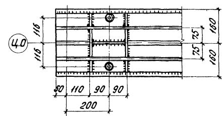
Разрез 3-3
