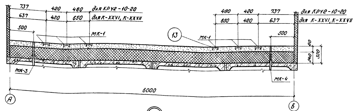
Разрез 1-1
