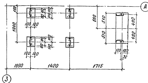
План фундаментов для лестницы у оси "А"
