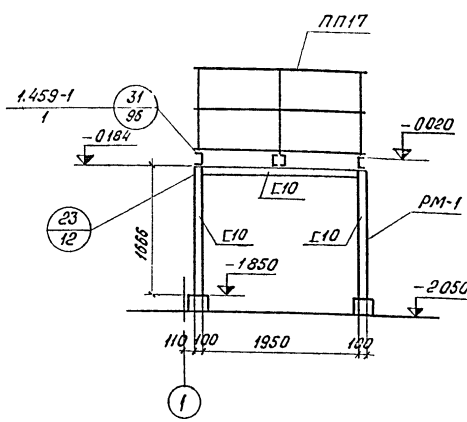
Вид 1-1
