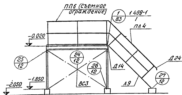
Вид 2-2
