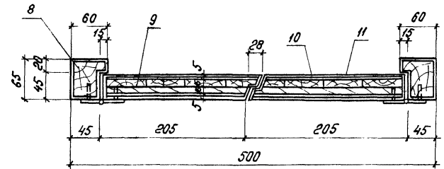
Разрез 3-3
