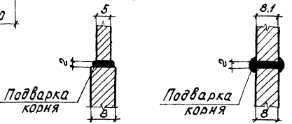
Сечение 6-6
