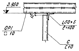
Вид 7-7
