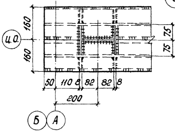
Сечение 6-6
