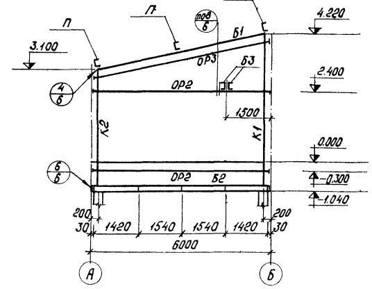
Вид 3-3
