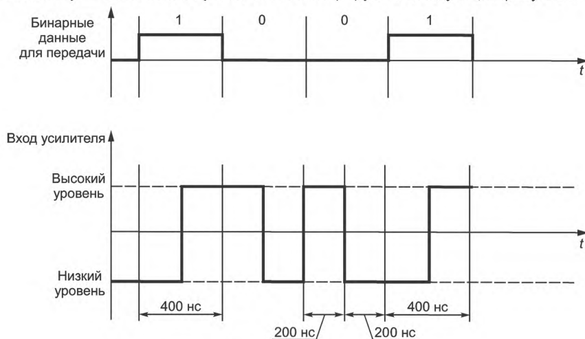
Рисунок 4 — Манчестерское кодирование
