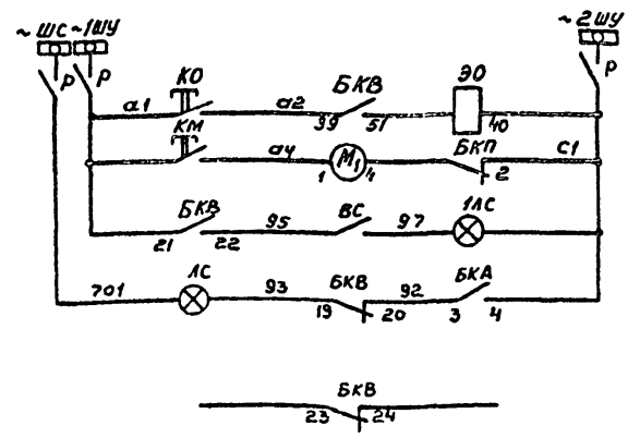
К тр-ру напряжения I секции шин
