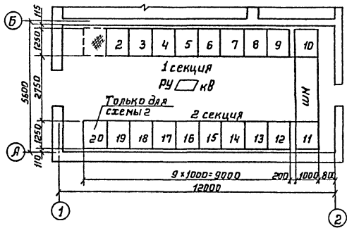
План РУ по схеме 3
