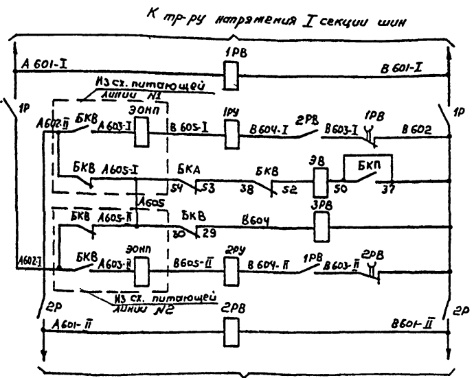
К тр-ру напряжения I секции шин
