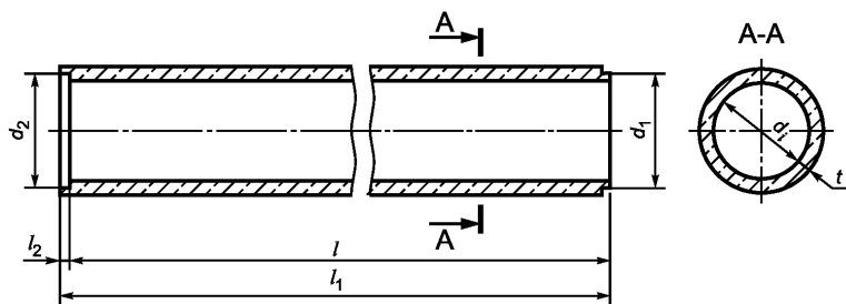
Рисунок А.3—Общий вид труб типа ТФ
