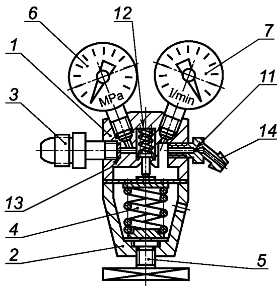
а) типовой редуктор с датчиком расхода
