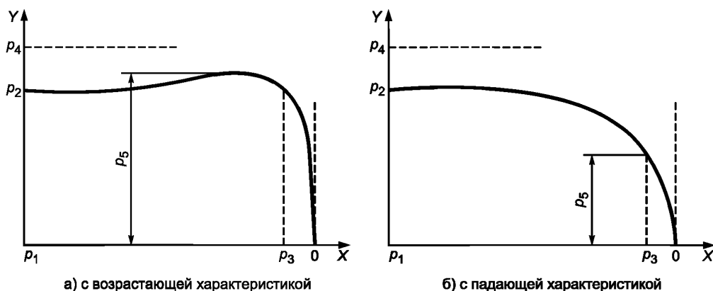
Рисунок 3 — Типовые динамические кривые расширения
