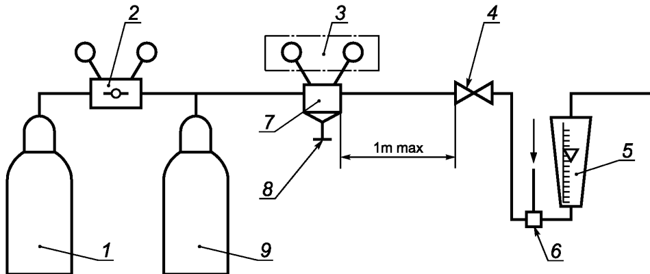
1 — источник газа; 2 — вспомогательный редуктор; 3 — калиброванные манометры; 4 — контрольный регулирующийся клапан; 5 — расходомер; 6 — термометр для измерения температуры газа; 7 — редуктор (испытуемый образец); 8 — задаточный винт; 9 — буферный баллон
