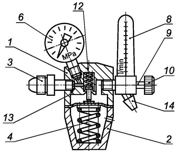
б) типовой редуктор с расходомером
