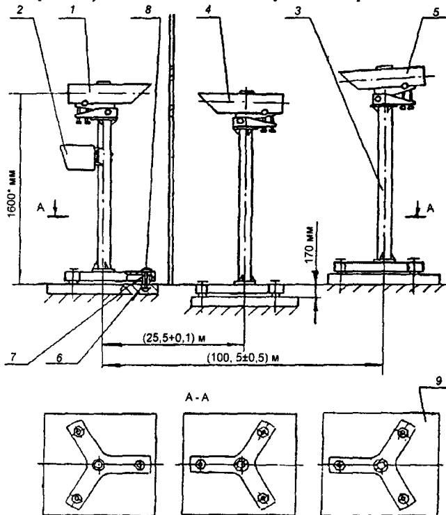
Рисунок А.8 — Схема расположения измерителя МОД на объекте
