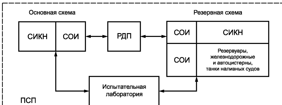
Типовая структурная схема ПСП
