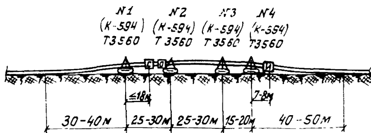
Рис. 9. Размещение механизмов в механизированной колонне при наземной прокладке трубопровода диаметром 1-20 м;
