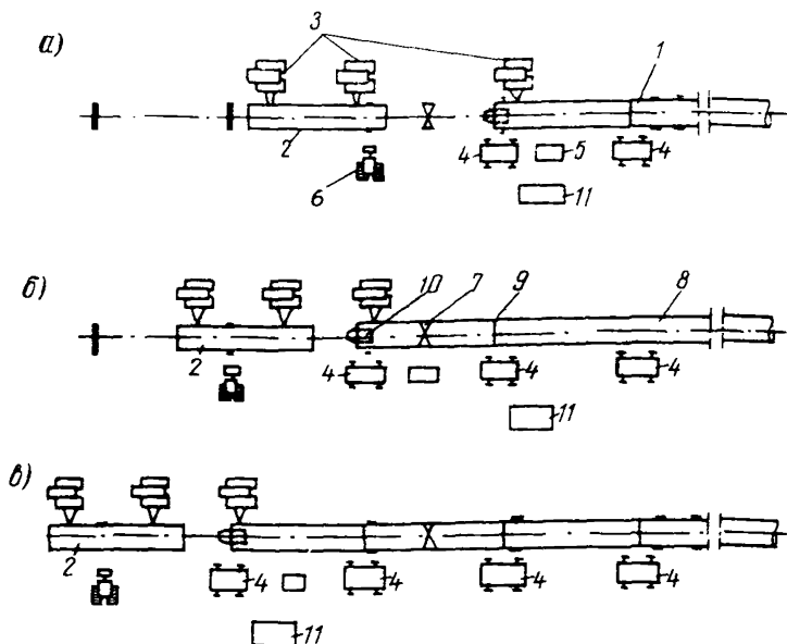
Рис.4. Монтаж прямолинейного участка надземного трубопровода: а - в-последовательность монтажа; I-смонтированный трубопровод; 2-собираемая секция; 3-трубоукладчики ТЗ560 или К-594; 4-сва- рочные агрегаты СДУ-2Б; 5-сани с кислородными и пропановыми баллонами; 6-бульдозер Д-271А; 7-неподвижная опора; 8-продоль- но-подвижная опора; 9-грунтовая или снежная призма; 10-центра- тор ЦВ-142 или ЦВ-141; II-передвижной домик
