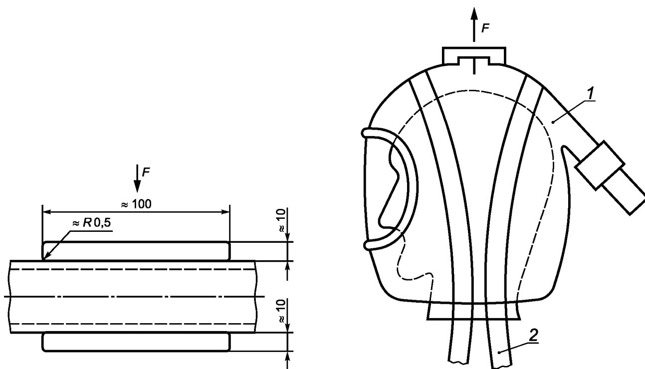
Рисунок 5 — Устройство для испытания сопротивления сжатия шланга подачи сжатого воздуха
