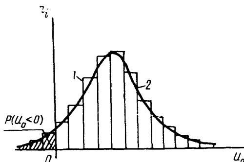
рис.10. Статистическое описание результатов вычисления (методом Монте-Карло) значений случайной величины \tilde{U}_0 (резерва прочности):
