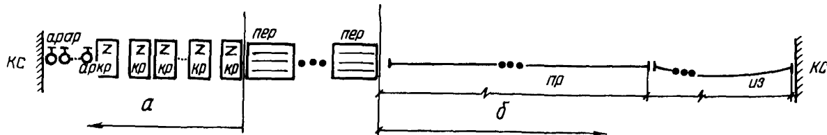
Рис.4. Условное представление структурной схемы надежности однопунктового газопровода (между двумя КС) как системы: а - совокупность последовательно соединенных протяженных (справа) и б - совокупность последовательно соединенных непротяженных (слева) элементов: пр - прямолинейный по проекту участок суммарной протяженности; из - уругоизогнутый по проекту участок суммарной протяженности; ар - элемент линейной арматуры; пер - переход через препятствие
