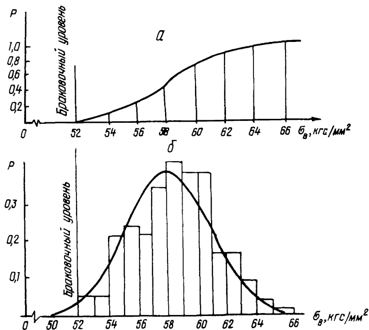
Рис.12. Пример описания кривыми Грама-Шарлье данных по временному сопротивлению \sigma_b труб диаметром 720х12 мм (для одной из марок сталей):
