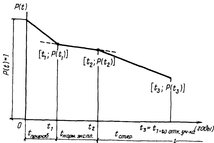
Рис.7. Кривая убыва надежности элемента линейной части до момента первого отказа линейного участка (между соседними Ю) в условиях допущения о пуассоновском (с переменным параметром) характере интенсивности отказа элемента
