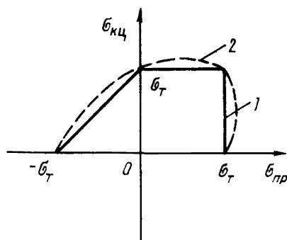
Рис.9. Допустимая область значений эквивалентных напряжений при действии внутреннего давления и продольных сил: 1—по критерию максимальных касательных напряжений; 2—по энергетическому критерию
