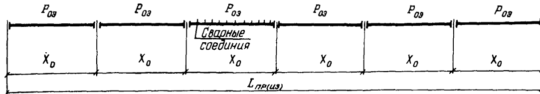
Рис.5. Расчетная модель протяженного прямолинейного (или уругоизогнутого) участка линейной части:
