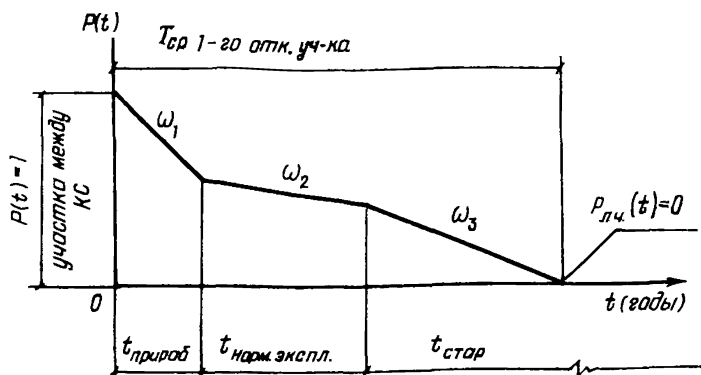
Рис.6. Кривая убывающей надежности расчетного участка линейной части (равного расстояния между соседними КС) в условиях допущения о пуассоновском (с переменным параметром) характере потока отказов
