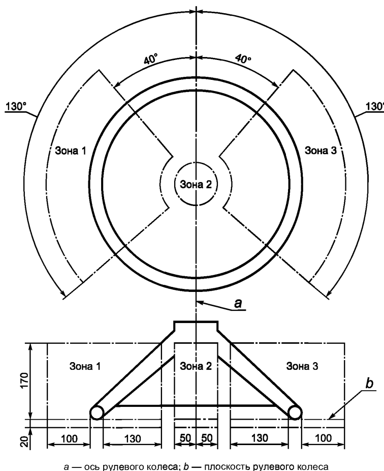
Рисунок 3 — Расположение зон
