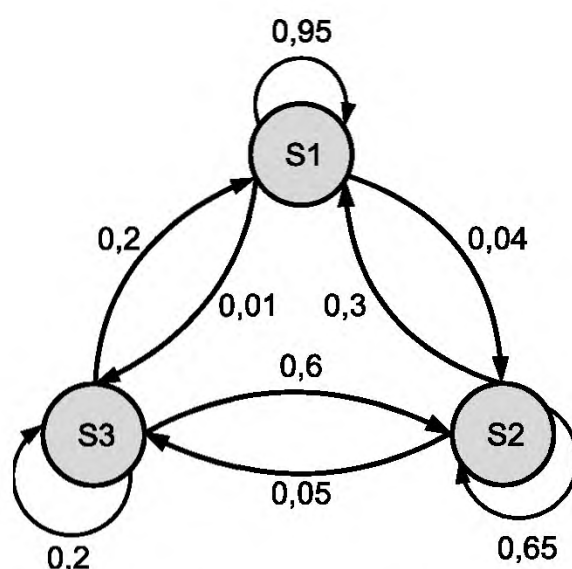
Рисунок В.9 — Пример диаграммы Маркова для системы
