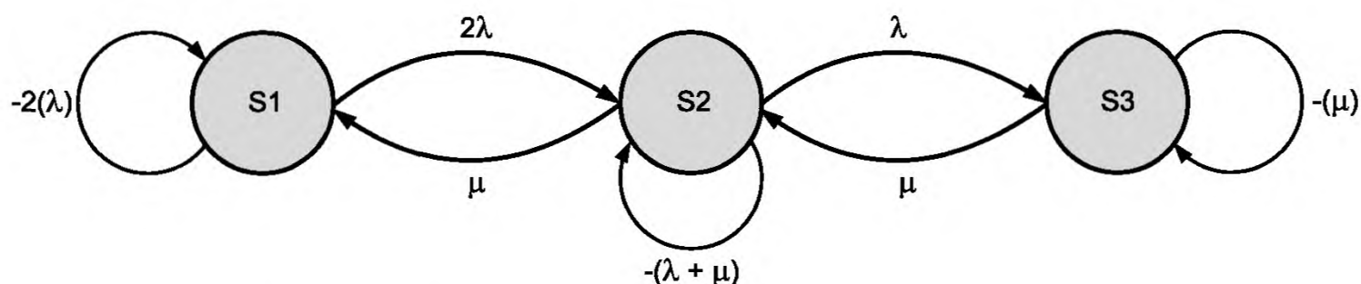
Рисунок В.10 — Пример диаграммы состояний перехода
