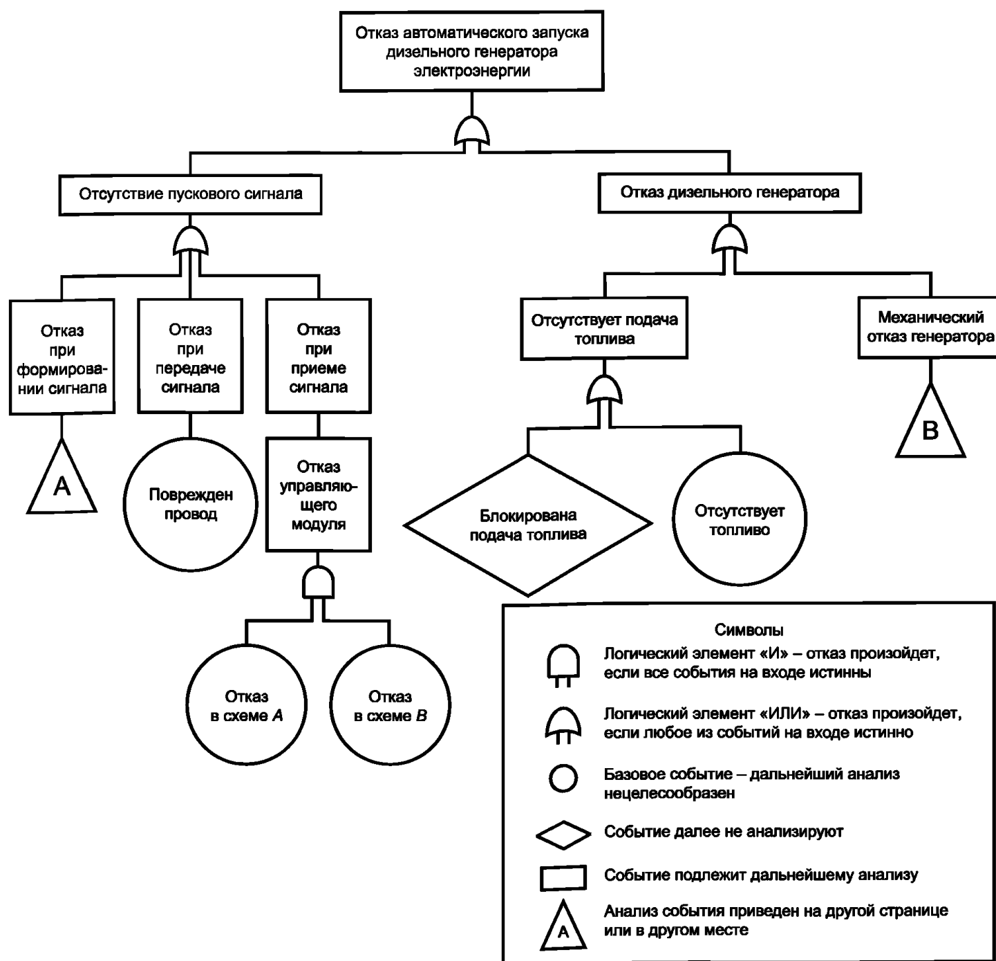
Рисунок В.2 — Пример метода FTA
