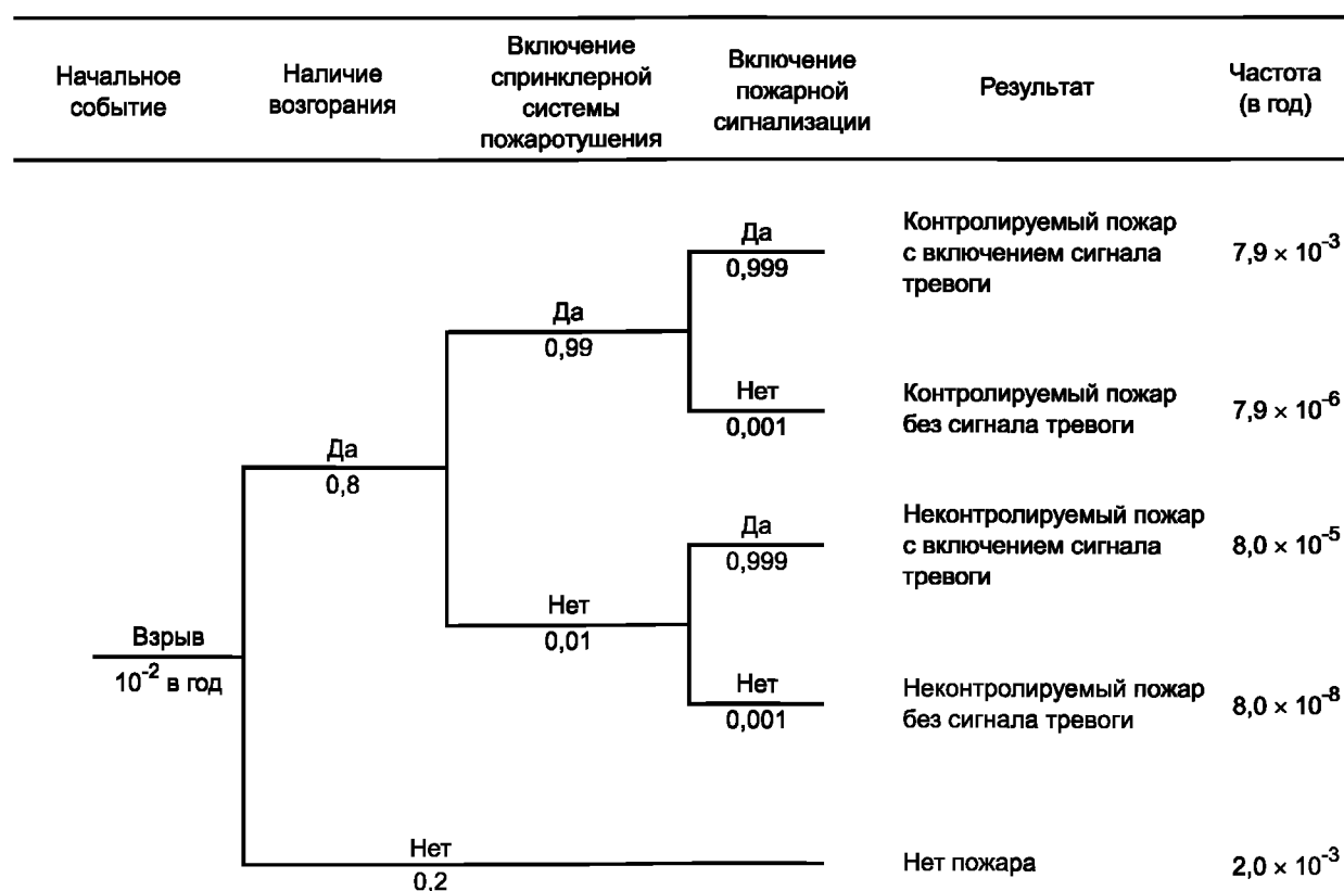
Рисунок В.3 — Пример дерева событий
