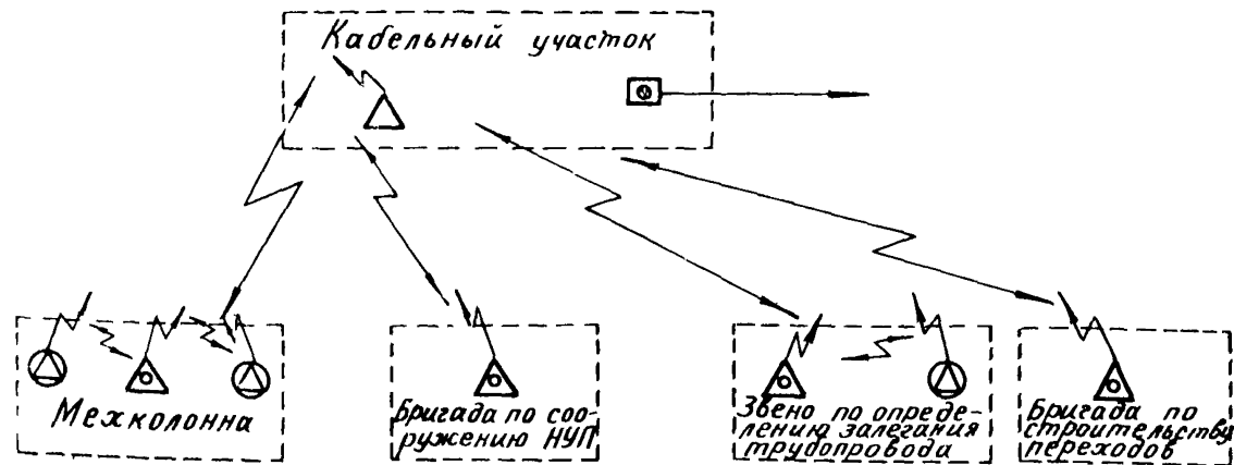
Рис.2. Схема организации радиосвязи кабельного участка: \triangle - радиостанция начальника кабельного участка; \triangle - мобильные УКВ радиостанции; \bigcirc - портативные УКВ радиостанции; \square - телефонный аппарат для выхода на сеть магистральной связи
