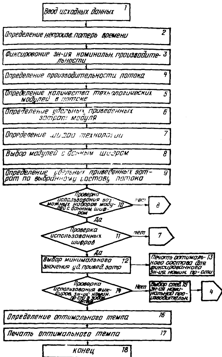
Рис.1. Блок-схема алгоритма расчета оптимального ресурсного состава и мощности потока
