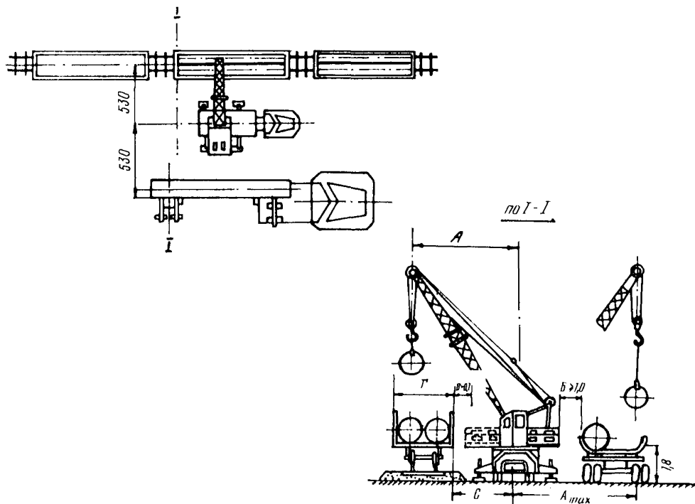
Рис. I. Схема выгрузки труб из полувагонов с погрузкой их на транспортные средства
