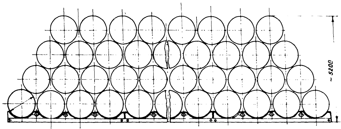
Рис.3. Сборно-разборный стеллаж СВ-1421
