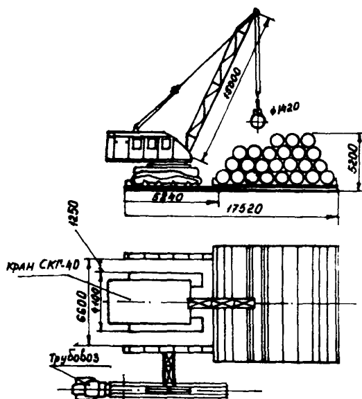
Рис.4. Схема складирования труб на стеллаж СР-1421 с помощью гусеничного крана СТ-40
