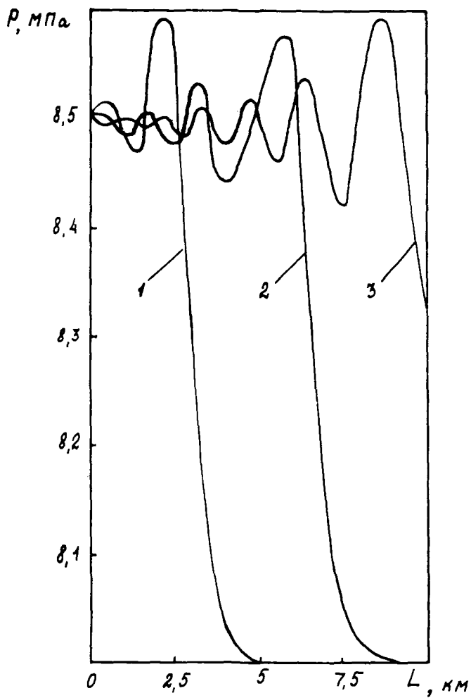
Рис.1. Кривые изменения давления жидкости ( P ) по длине трубопровода ( L ) в различные моменты времени ( t ):
